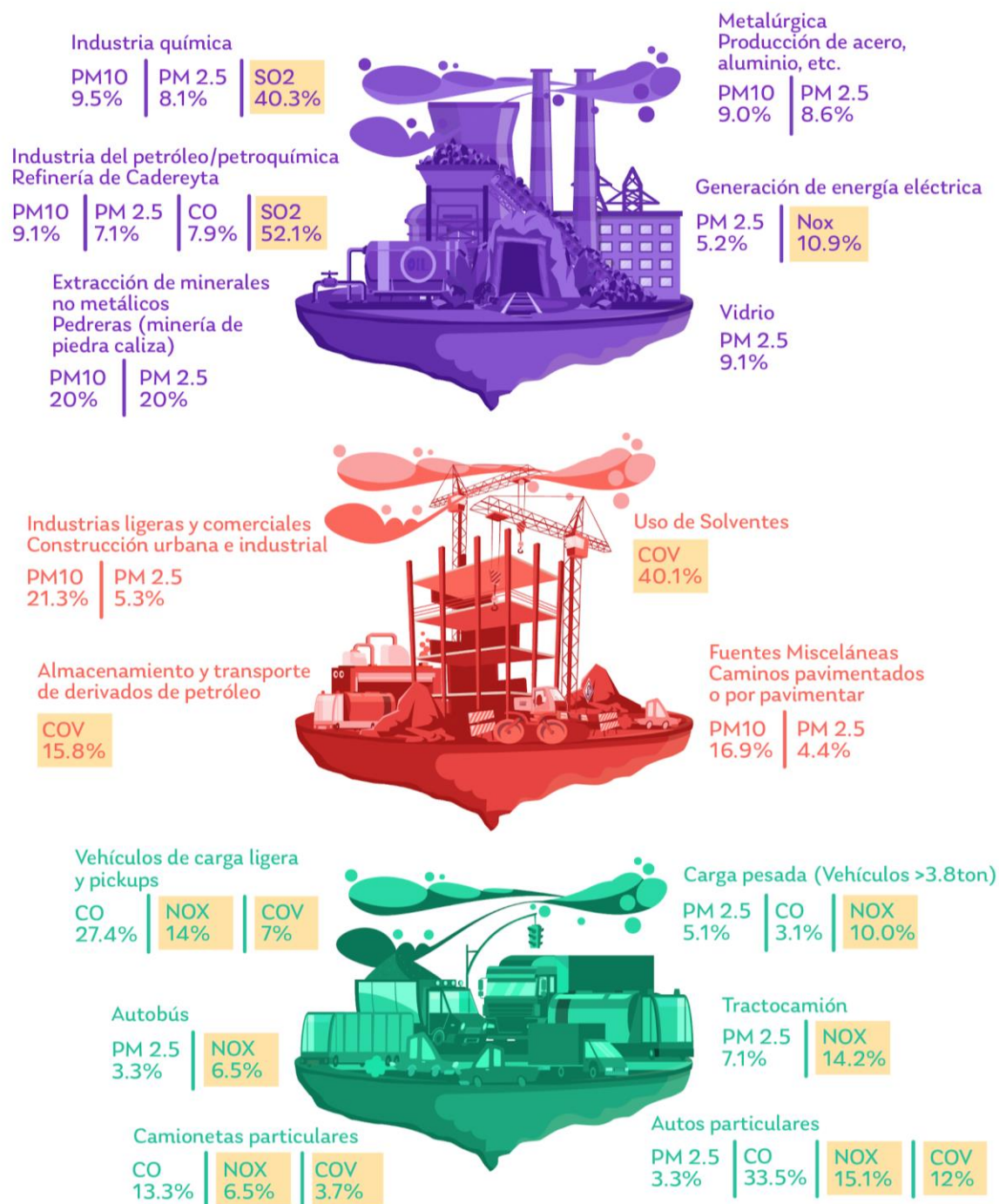
Figura 2. Porcentaje de aportación al total de emisiones de cada contaminante por actividad económica e industria en Nuevo León
